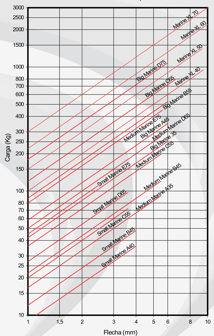
CURVA DE CARGA FLECHA AMC MECANOCAUCHO® Tipo MARINO
